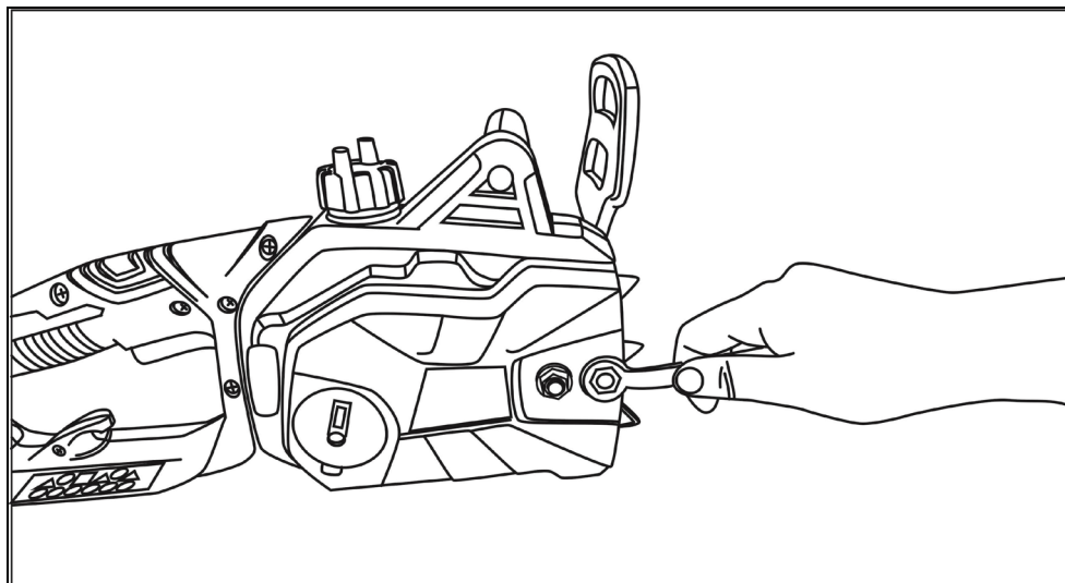
Рис. 1. Откручивание крепежного винта шины
