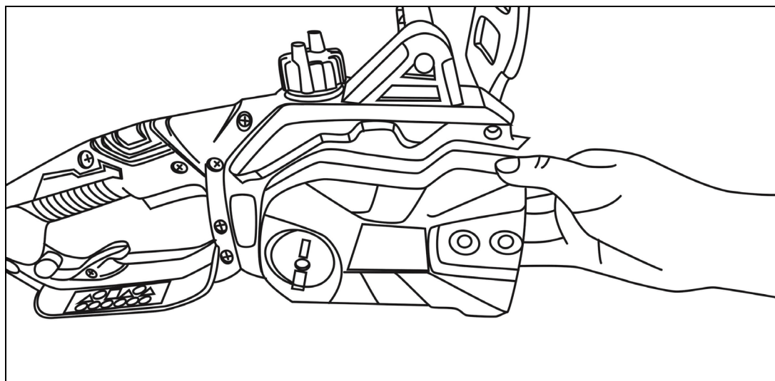
Рис. 2. Снятие прижимной крышки шины
