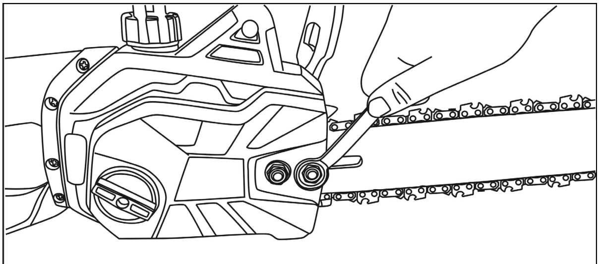
Рис. 4. Фиксация шины прижимной крышкой
