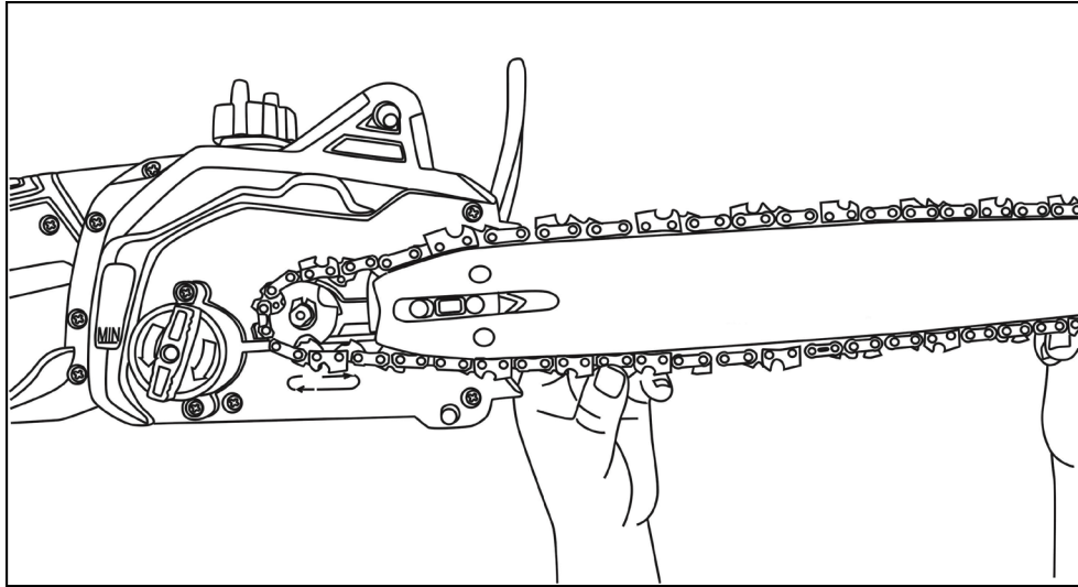
Рис. 3. Установка шины и цепи
