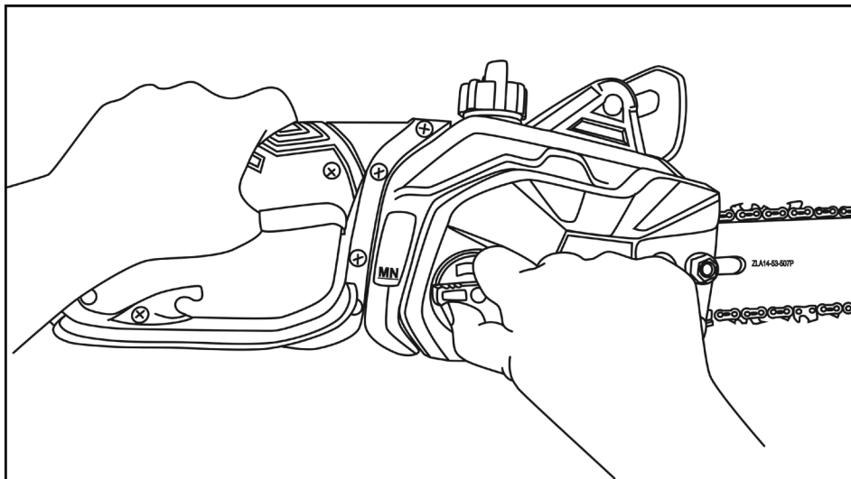
Рис. 5. Натяжение цепи винтом натяжителя
