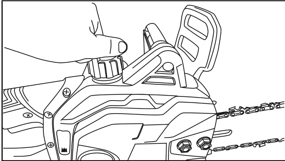
Рис. 7. Откручивание крышки маслоналивной горловины
